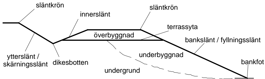
Figur b Vägkonstruktion (VVFS 2007:103)
